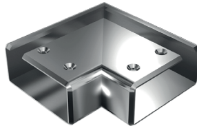
60x25 90° Dirsek Önden Kanallı 60x25 90° Elbow Front Channel
